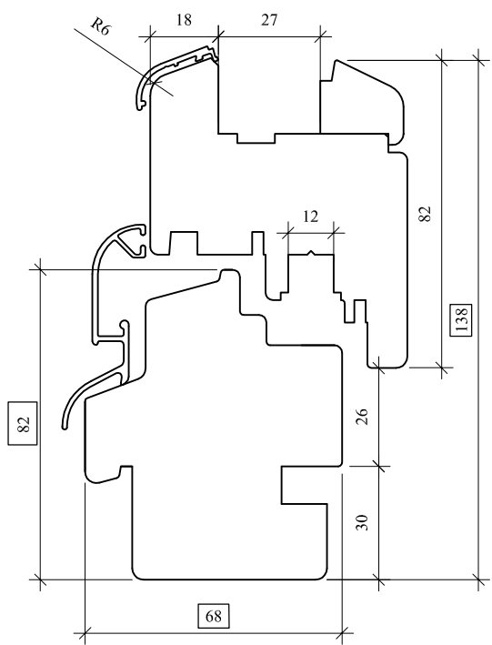
RAAM PROFIEL 68
