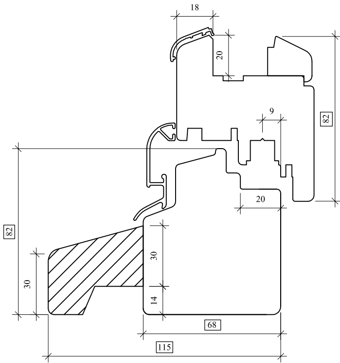
HOUT RAAM PROFIEL 68 NL
